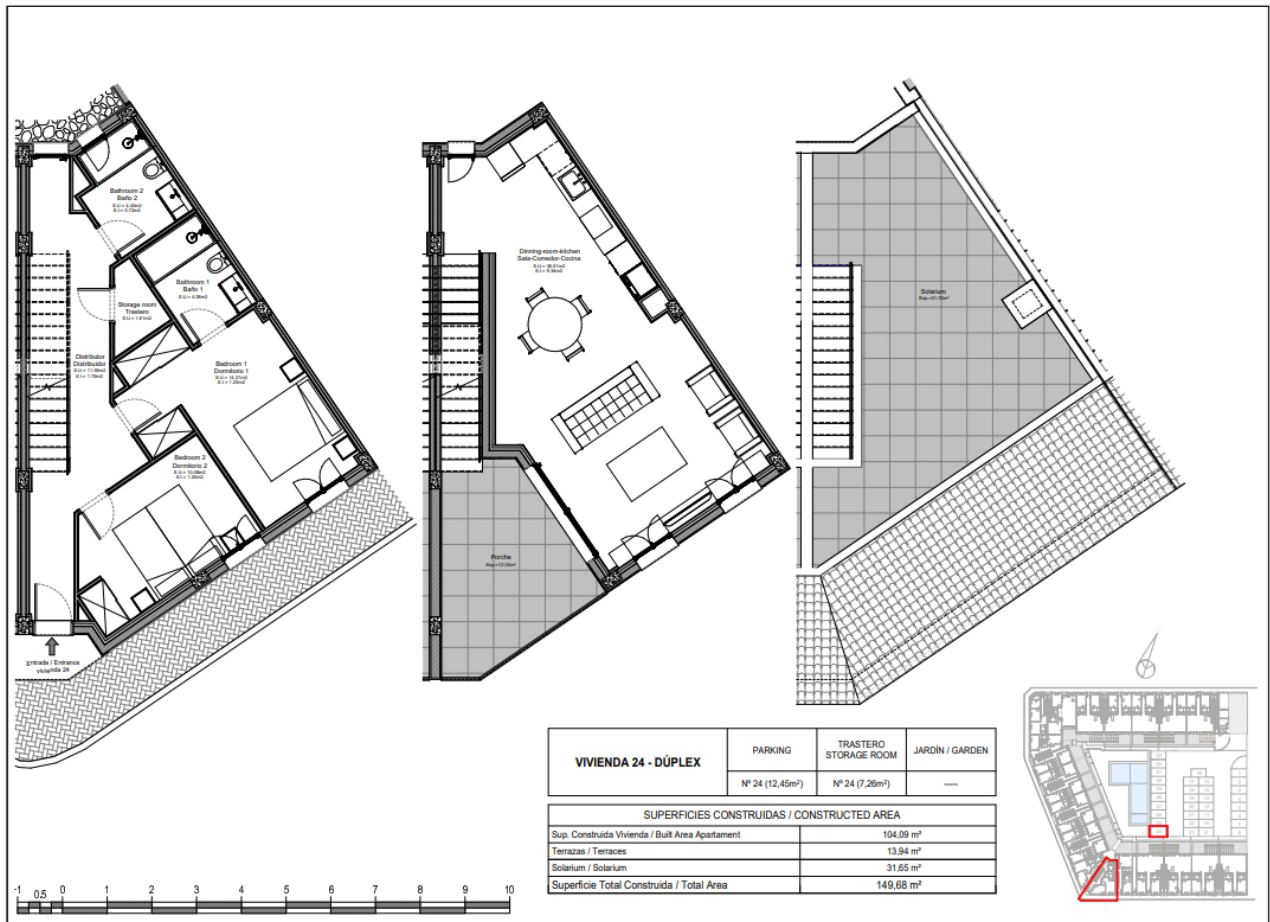
Plano B1-DU-24
