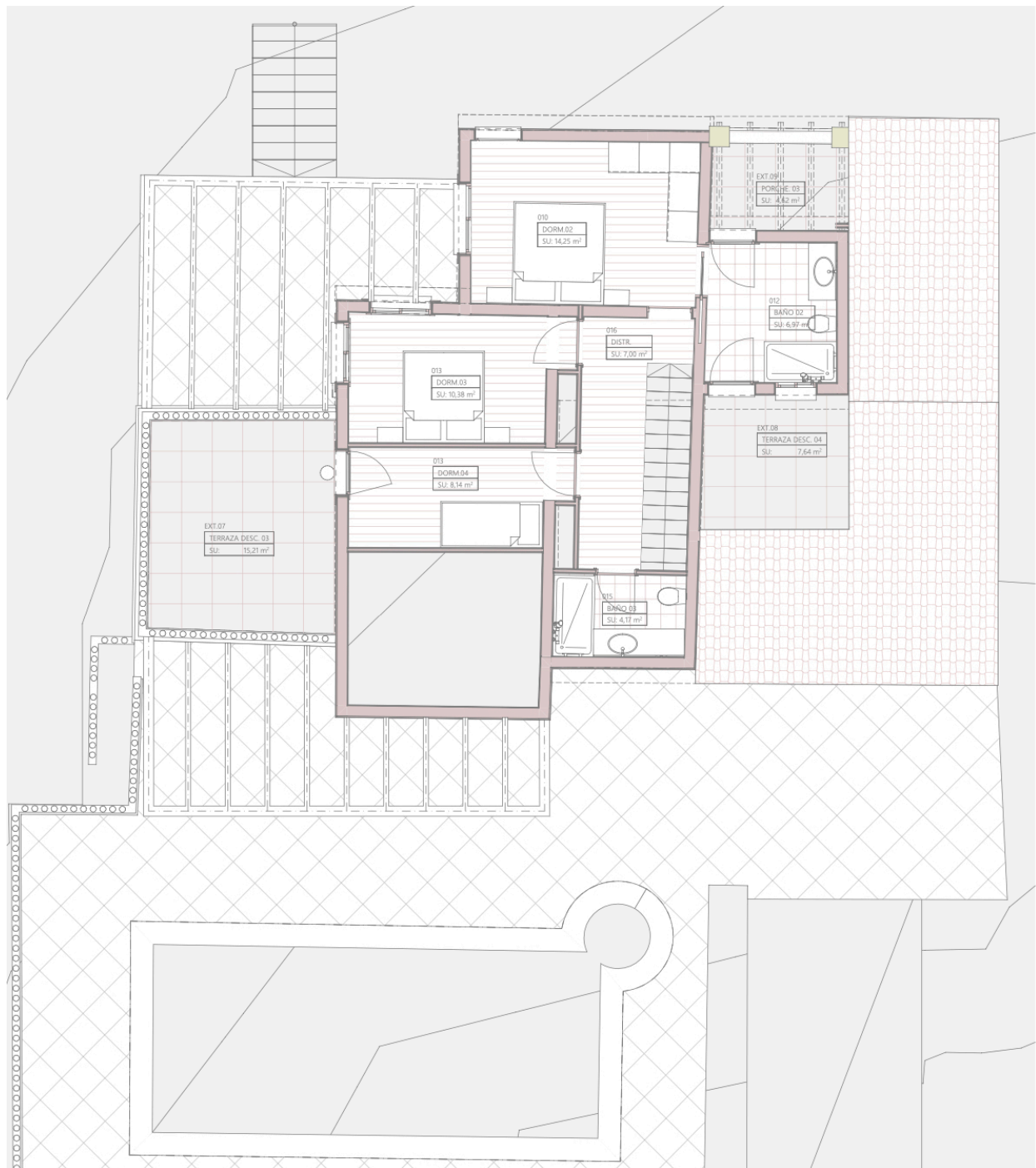
Grundriss Obergeschoss
