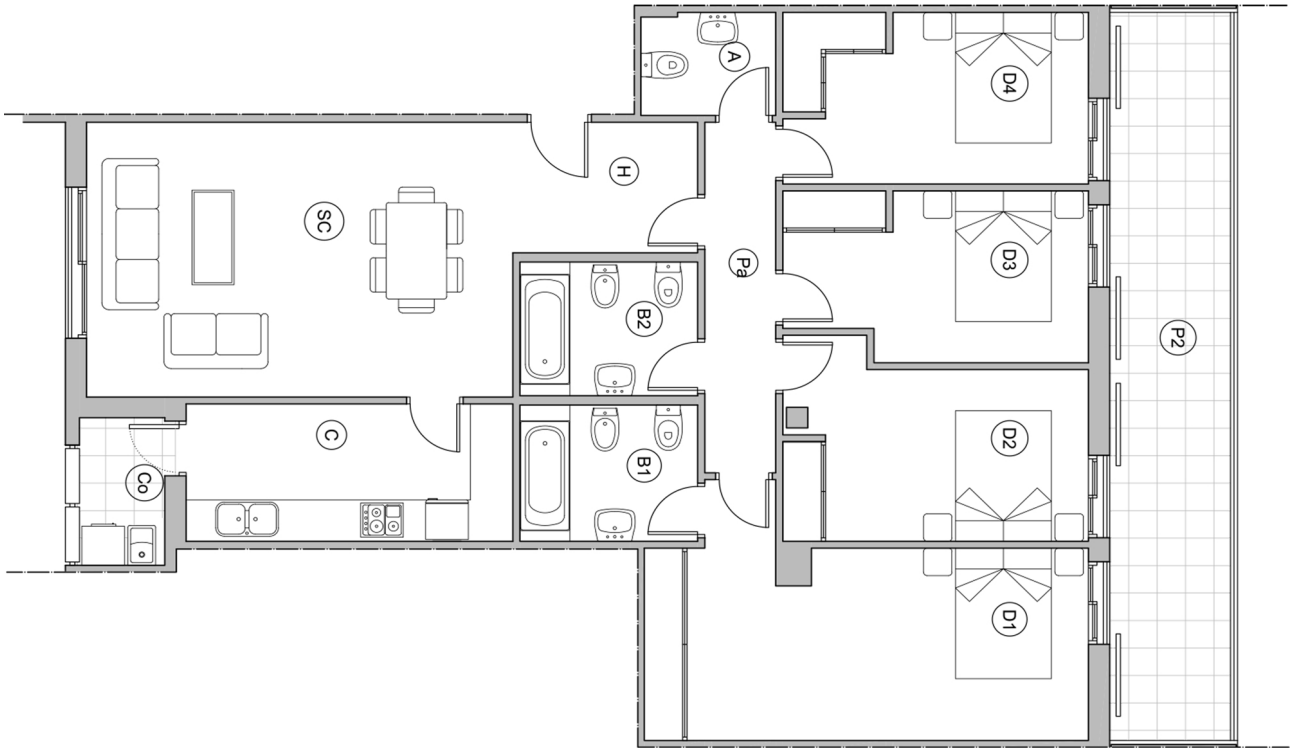
Grundriss
