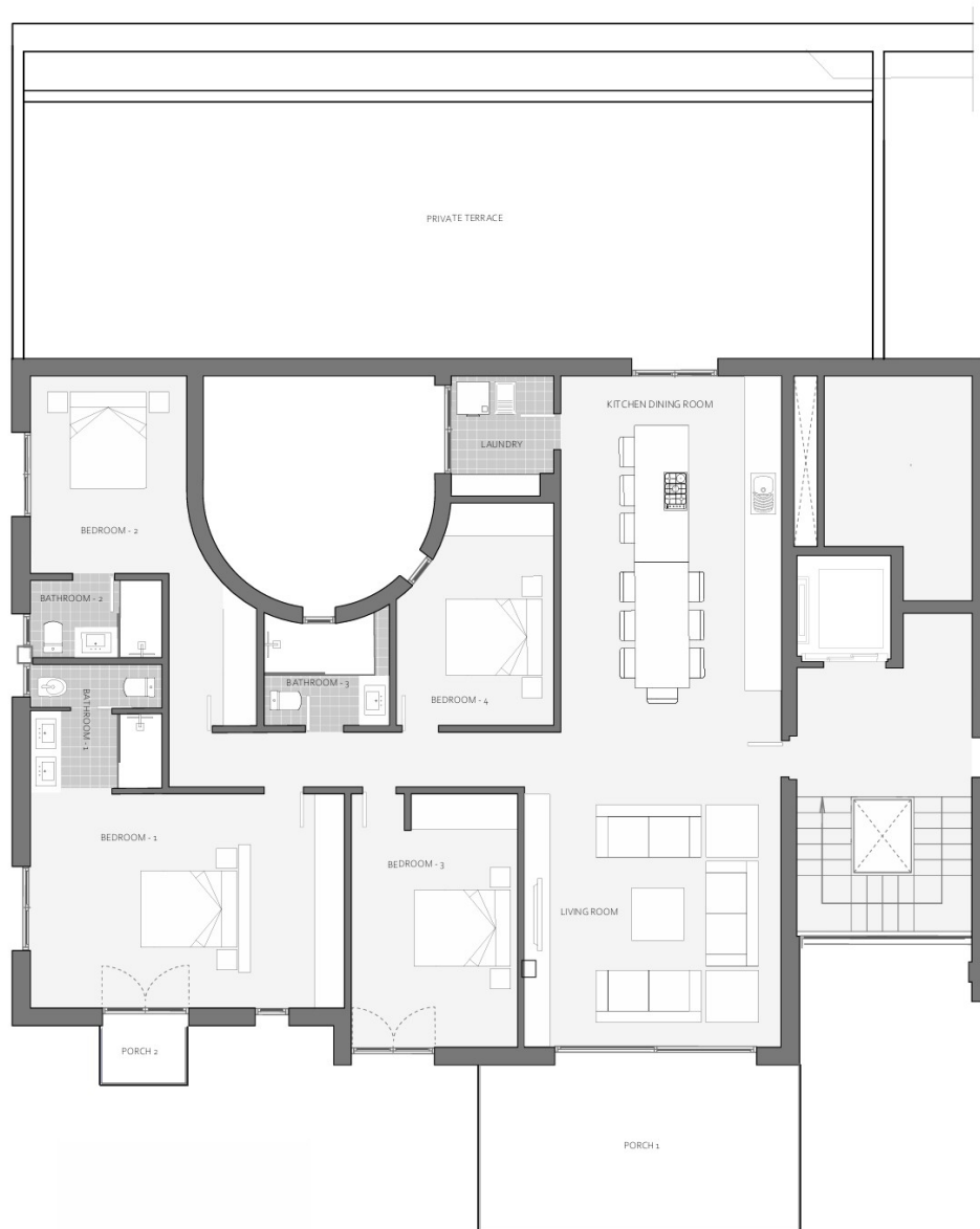
Plano Planta 3
