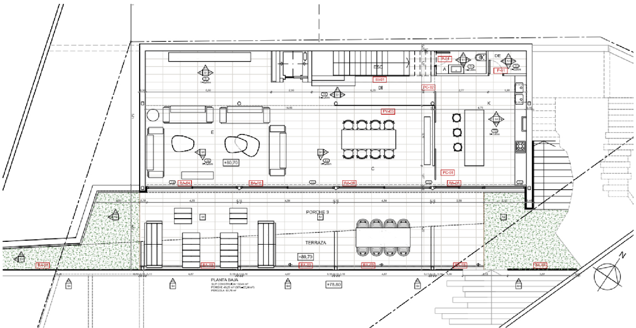
Grundriss - EG
