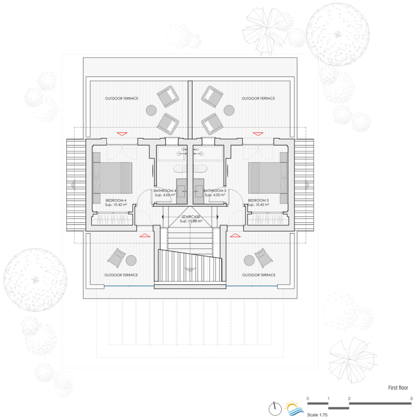
Grundriss Obergeschoss
