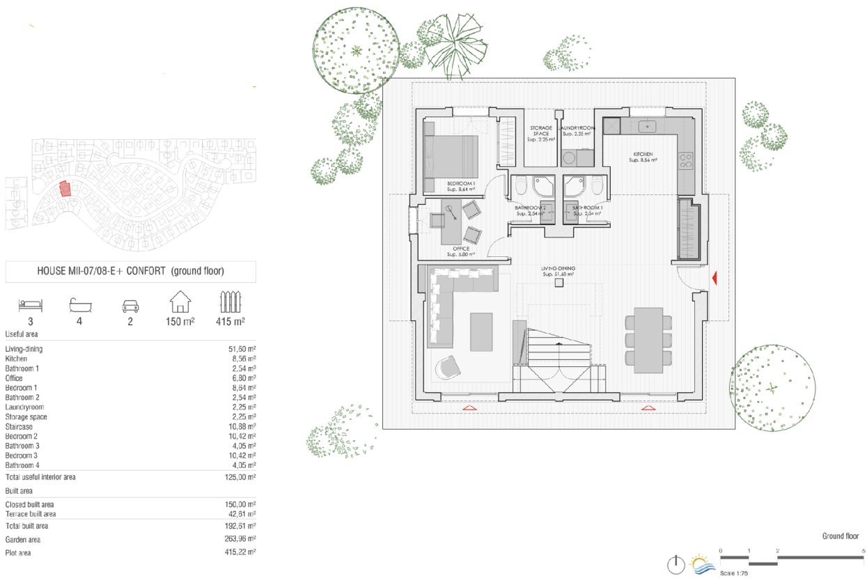
Plano MII-07-08-E+ (Planta Baja)
