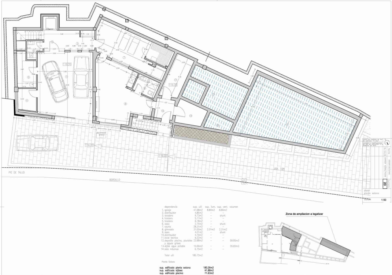
Plano Sotano
