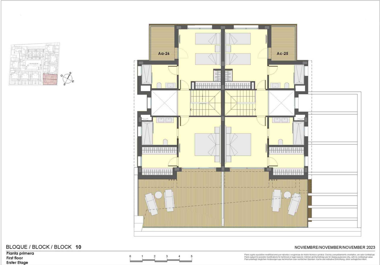
Plano Casa 26 (Planta Piso)
